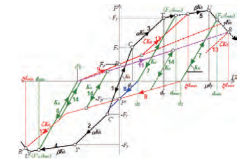
負勾配・耐力低下・ピンチング効果を表現した木造用の復元力特性
