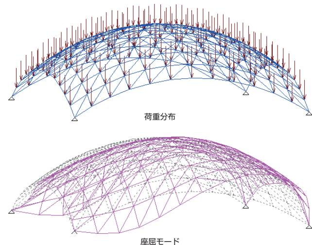
座屈モード
