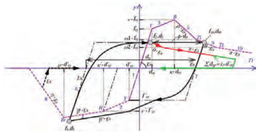
局部座屈を表現したMSモデル用の復元力特性
