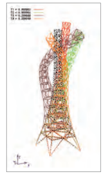
部材レベルの固有モード図
