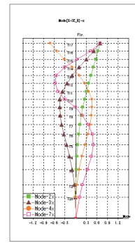
層レベルの固有モード図
