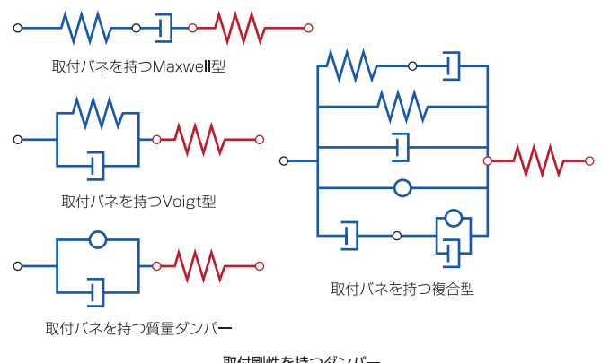
取付剛性を持つダンパー
