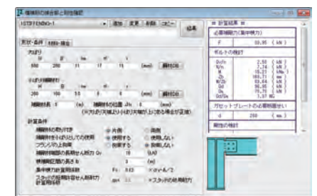
横補剛の接合部と剛性確認
