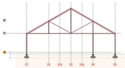
山形トラス(フレーム図)
