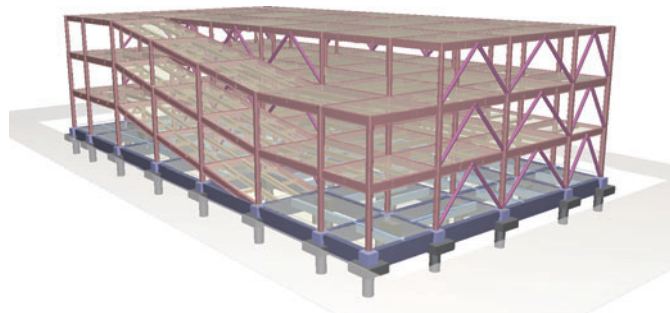
自走式駐車場
