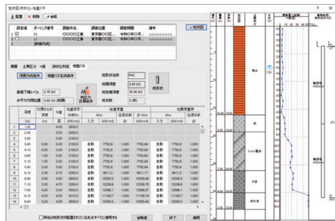
地盤バネダイアログ
