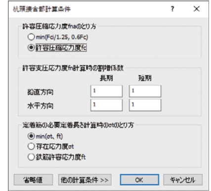
杭頭接合部計算条件ダイアログ
