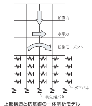
上部構造と杭基礎の一体解析モデル
