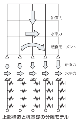
上部構造と杭基礎の分離モデル
