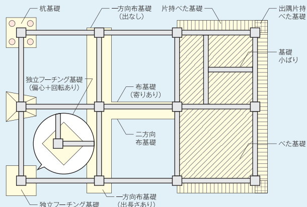
扱う基礎の形状
