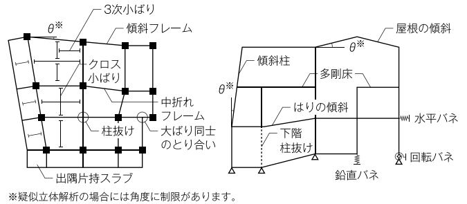
図1 平面図
